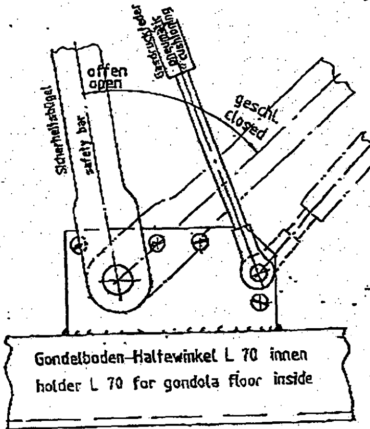
Zusammenbau Assembly Sc: 1.2
